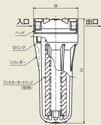
●構造図：NFH-NPP/-A/-H
